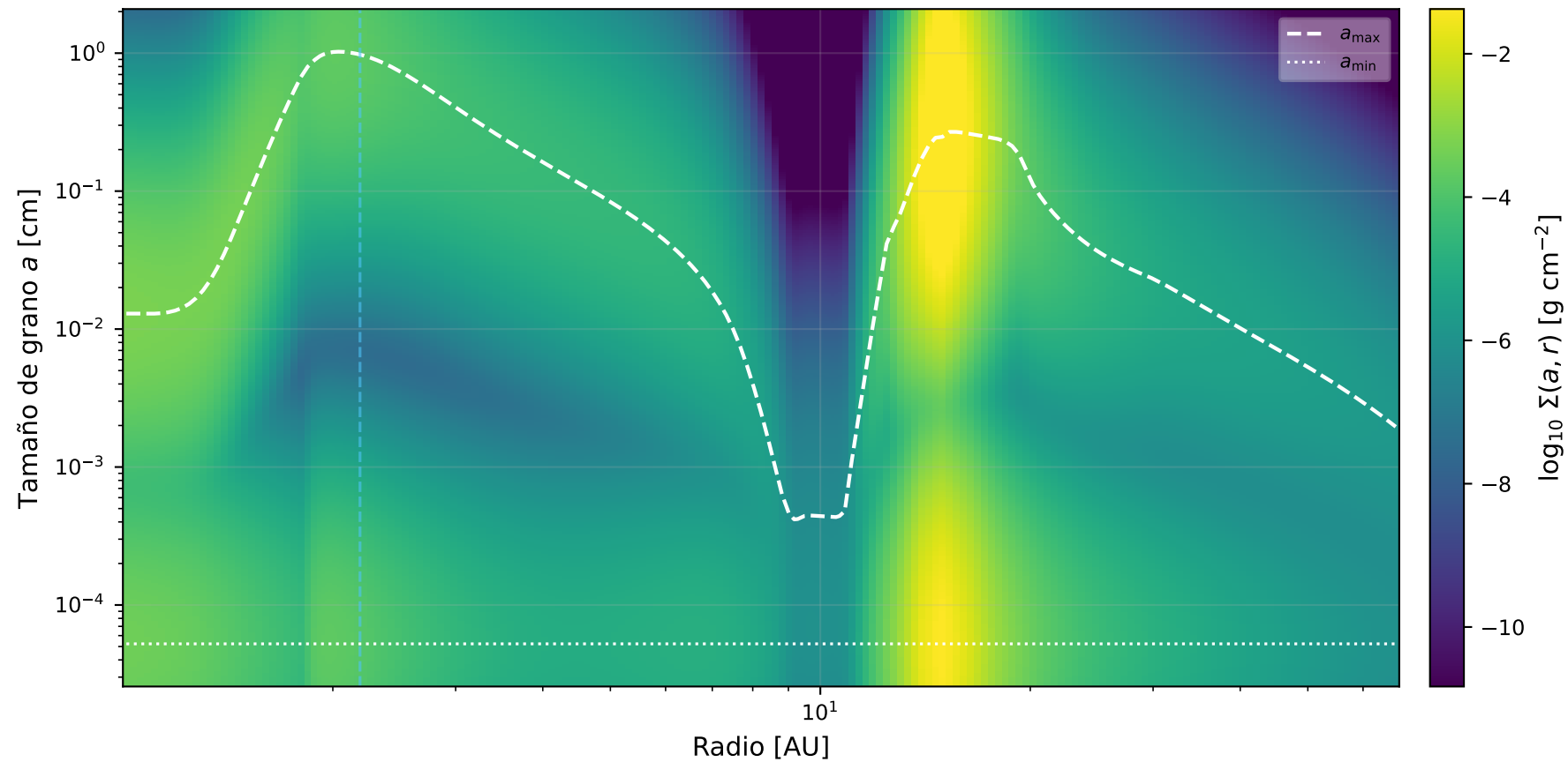
Distribución de tamaño de grano vs radio | t = 5.00\text{e}+06 yr
